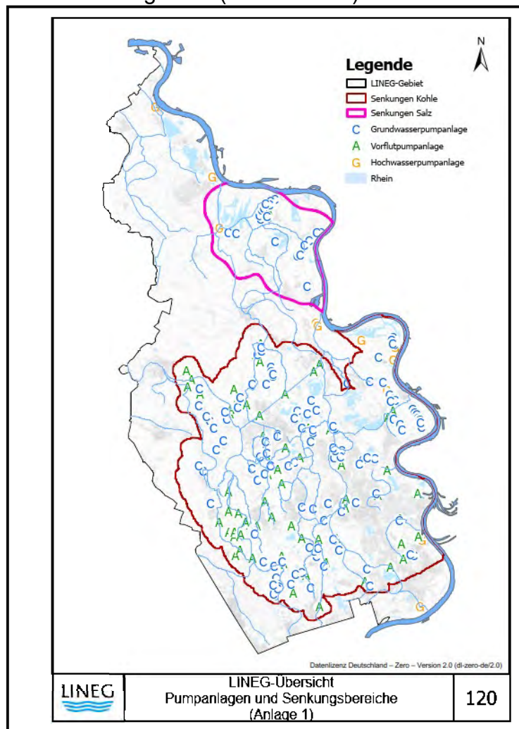
Abbildung 1: Senkungsbereiche und Wasserhaltungsmaßnahmen im LINEG-Gebiet
