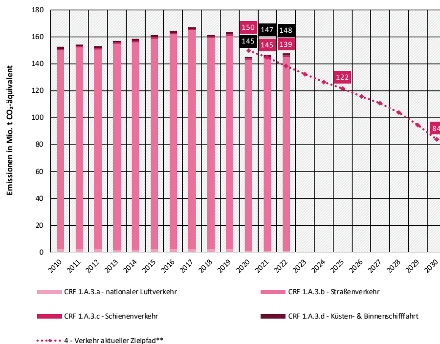
Abbildung 5: Entwicklung und Zielerreichung der Treibhausgas-Emissionen in Deutschland im Sektor Verkehr des Klimaschutzgesetzes (KSG)
