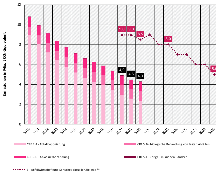
Abbildungung 7: Entwicklung und Zielerreichung der Treibhausgas-Emissionen in Deutschland - im Sektor Abfallwirtschaft und Sonstiges des Klimaschutzgesetzes (KSG)
