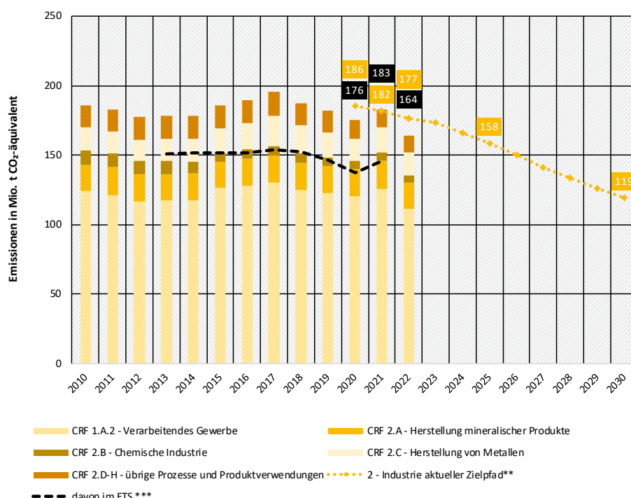
Abbildung 3: Entwicklung und Zielerreichung der Treibhausgas-Emissionen in Deutschland im Sektor Industrie des Klimaschutzgesetzes (KSG) 2
