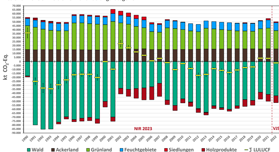
Emissionen LULUCF: Zeitreihen Landnutzungskategorien
